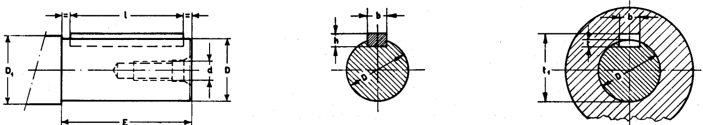
Langsamlaufende Hohlwelle Hollow low speed shaft Arbre lent creux
